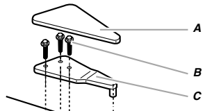
A. Couverture de la charnière supérieure B. Vis de charnière à tête hexagonale de 5/16"
